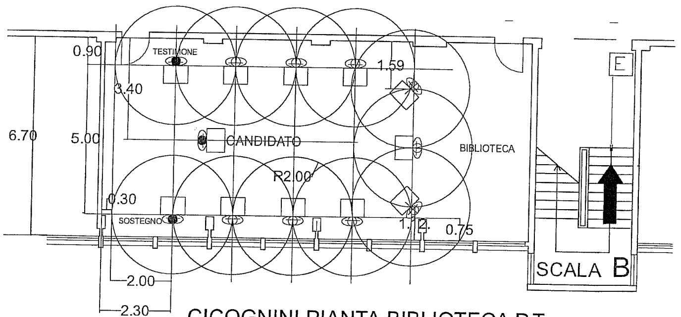
CICOGNINI PIANTA BIBLIOTECA P.T.
